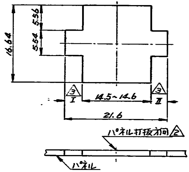
取付穴寸法(寸法公差±0.1) 尺度 Z-1
